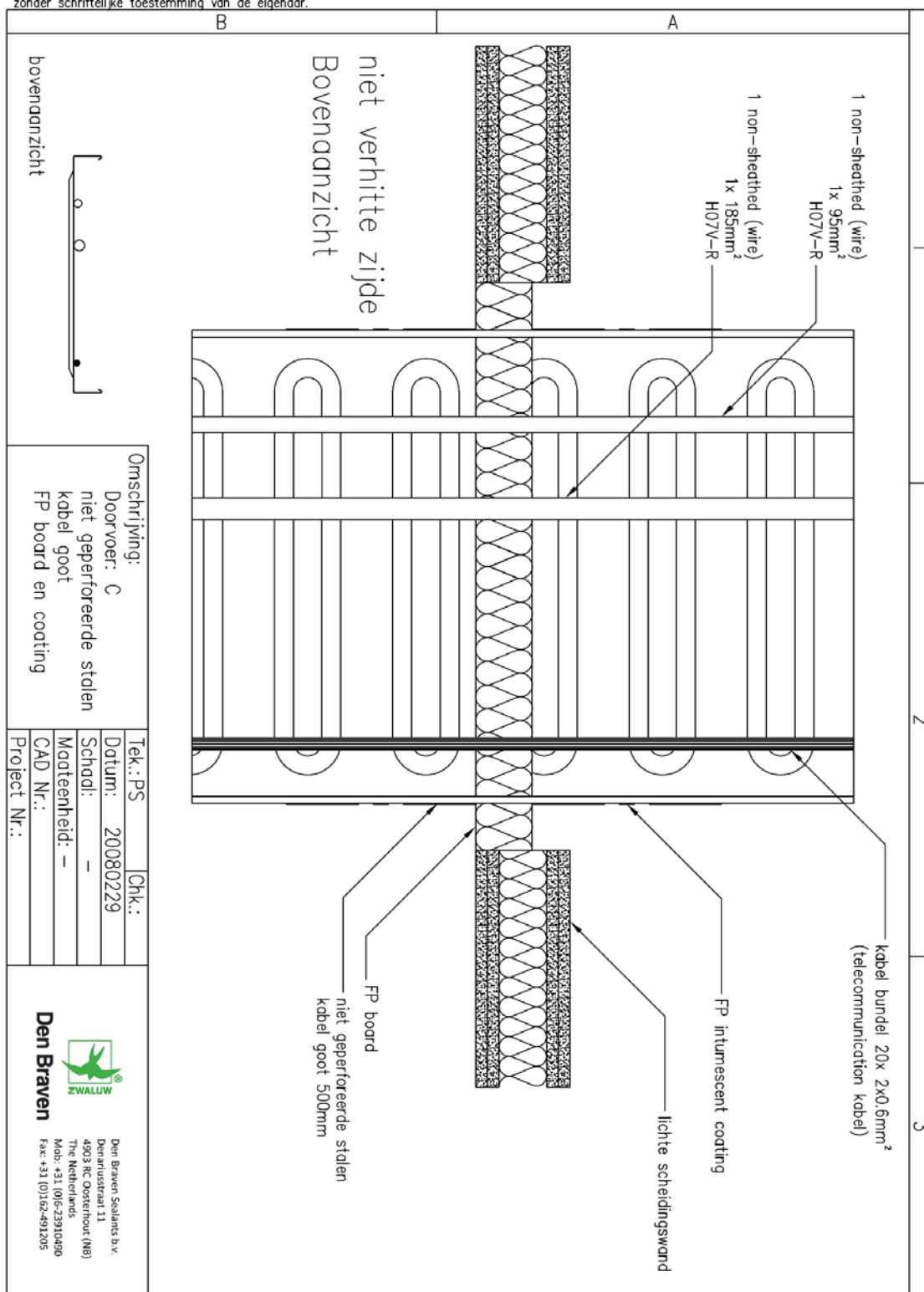
Figuur 24. Detail proefstuk C d.d. 06-06-2008, gebaseerd op 2008-Efectis-R0451
