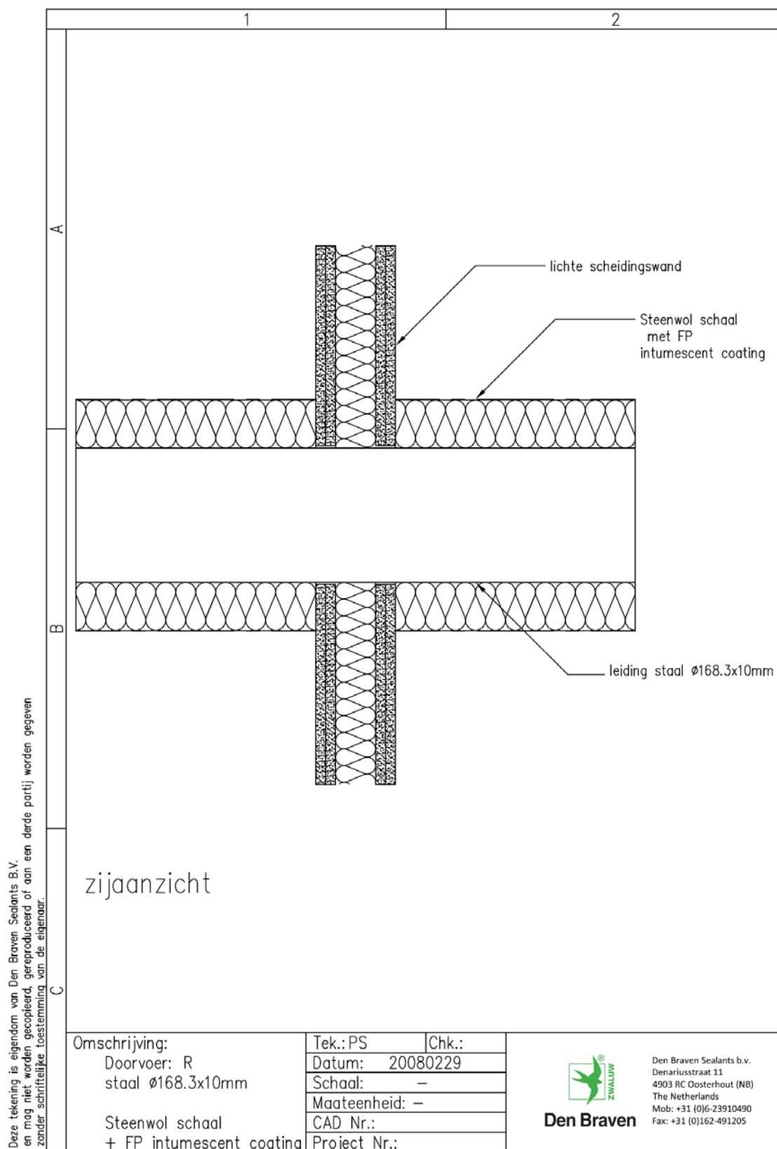
Figuur 31. Detail proefstuk R, gebaseerd op 2008-Efectis-R0456[Rev.1]
