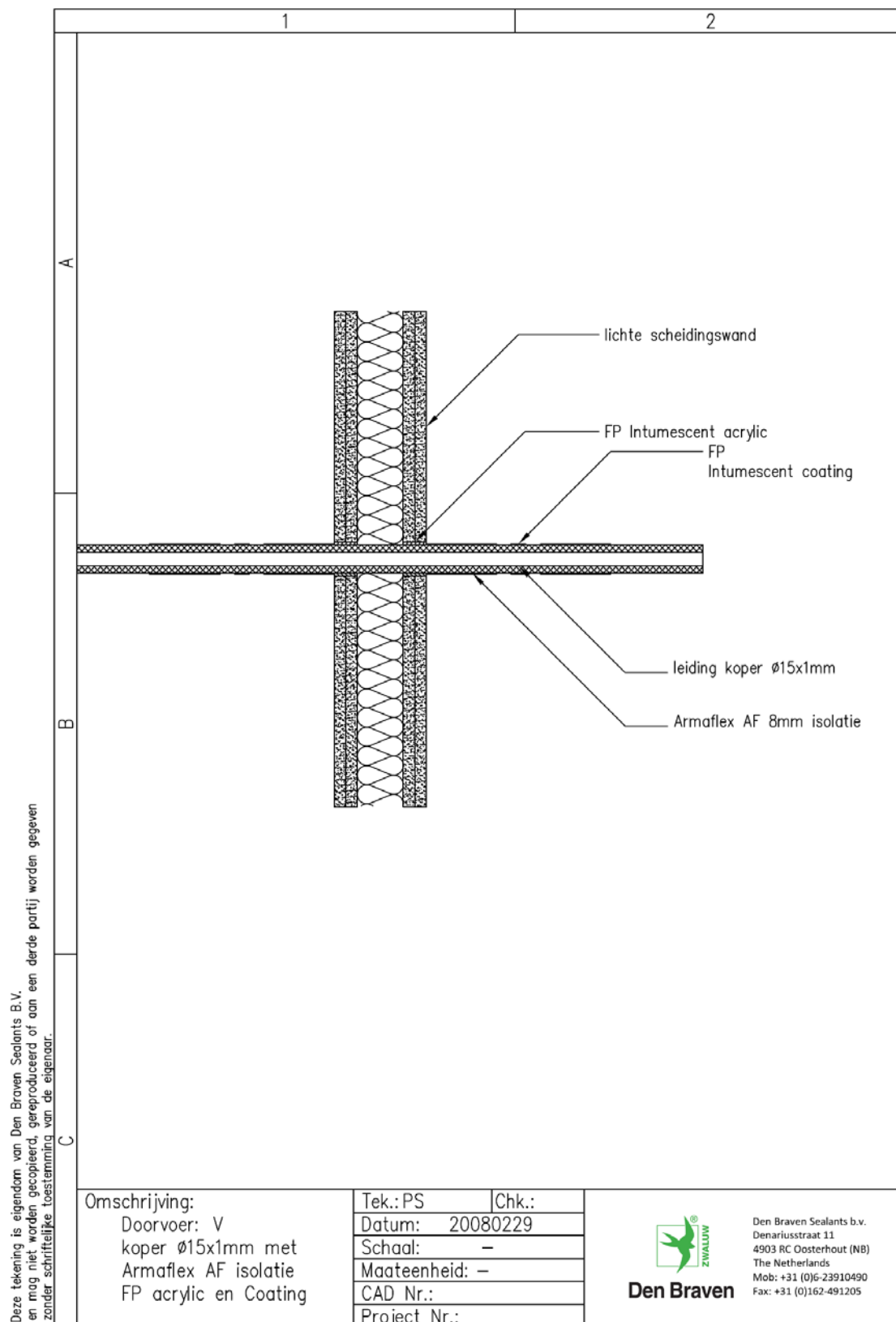
Figuur 34. Detail proefstuk V, gebaseerd op 2008-Efectis-R0457[Rev.2]
