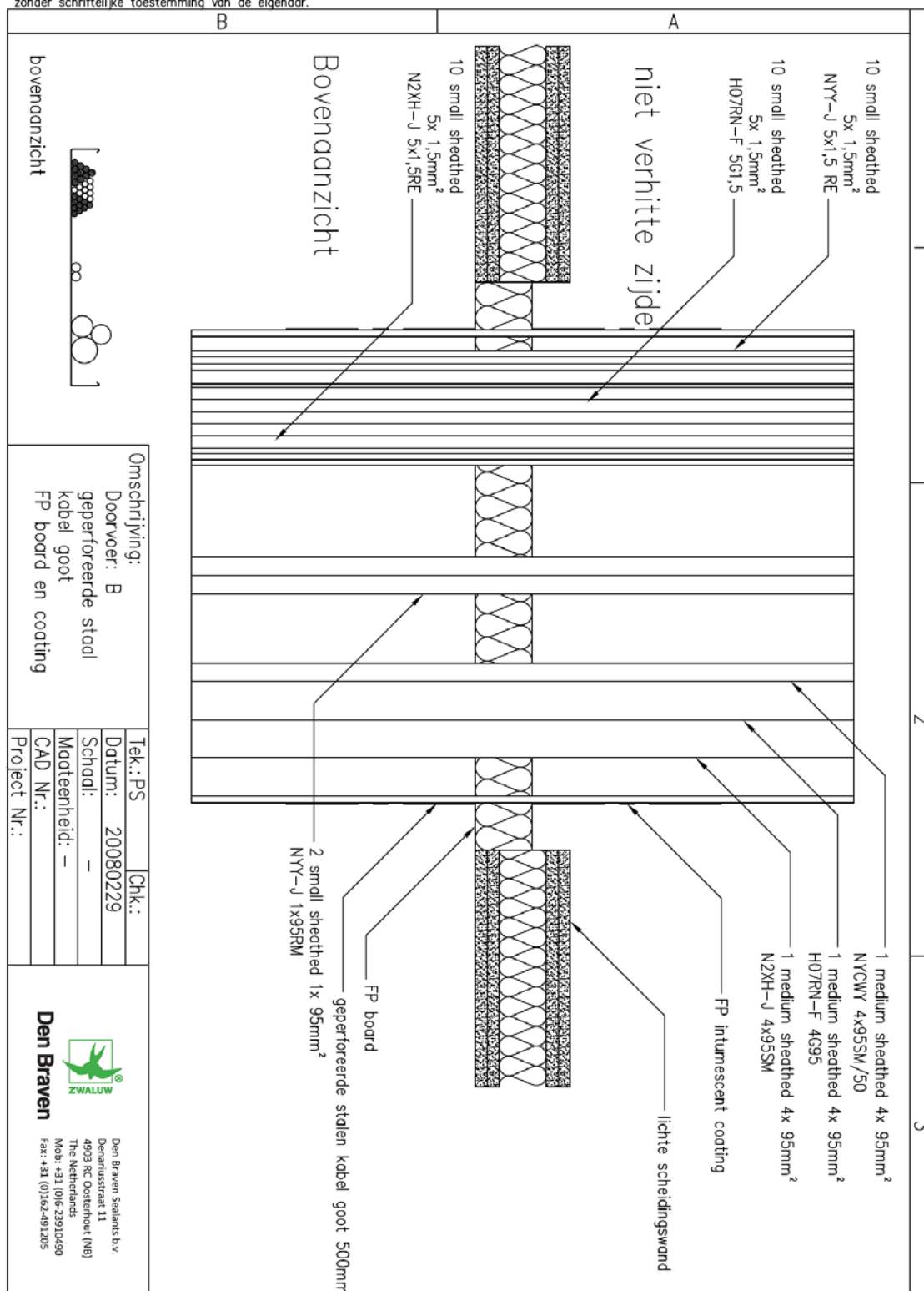
Figuur 19. Detail proefstuk B d.d. 27-03-2008, gebaseerd op 2008-Efectis-R0451
