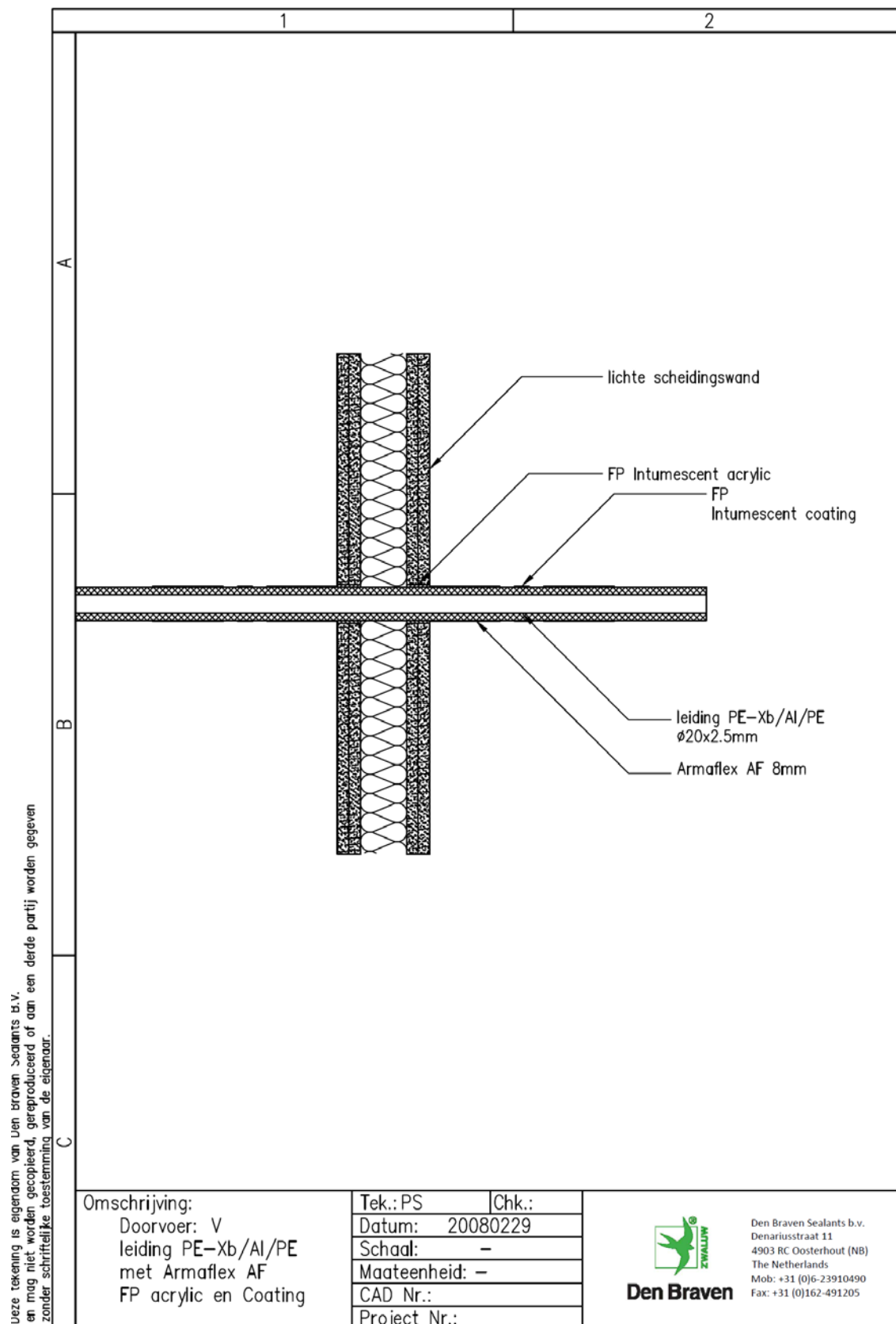
Figuur 39. Detail proefstuk V, gebaseerd op 2008-Efectis-R0461[Rev.1]
