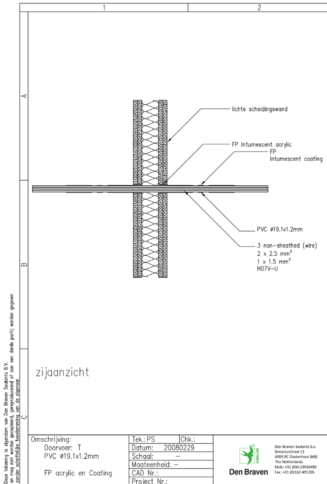
Figuur 35. Detail proefstuk T, gebaseerd op 2008-Efectis-R0458[Rev.2]
